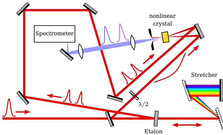
Bsp. 11.33: Angepasst von DOI:10.1364/AOP.1.000308, Abb. 37
