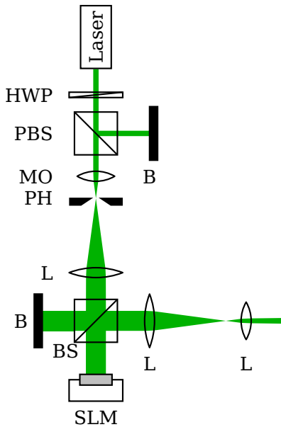
Bsp. 11.6: Angepasst von arXiv:1112.5270v2
