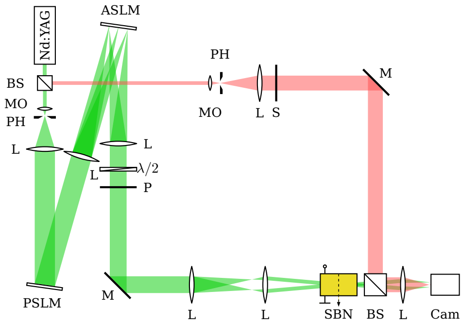
Bsp. 11.32: Angepasst von DOI:10.1364/OL.37.000797
