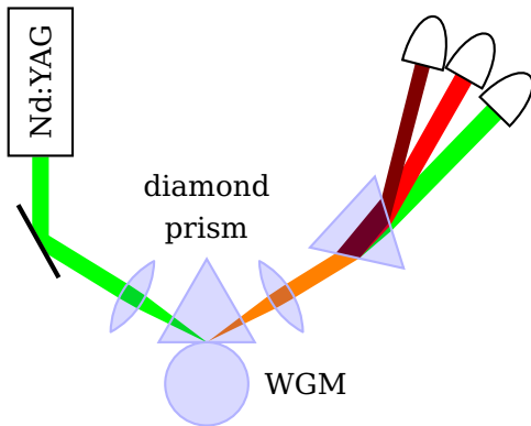
Bsp. 11.27: Angepasst von DOI:10.1103/PhysRevLett.105.263904
