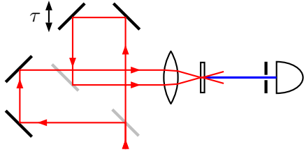
Bsp. 11.25: Angepasst von DOI:10.1364/AOP.1.000308, Abb. 8
