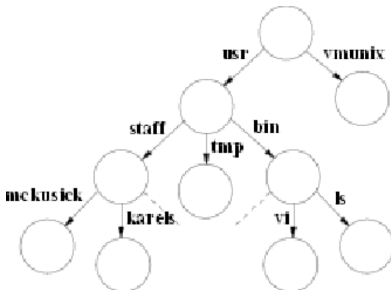
図2.2 小規模なファイルシステム
